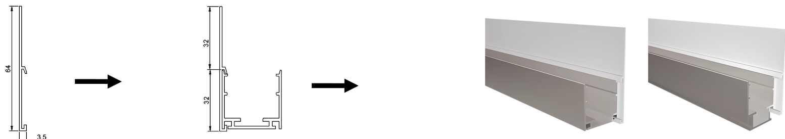
Shading plate : 7012721-05
