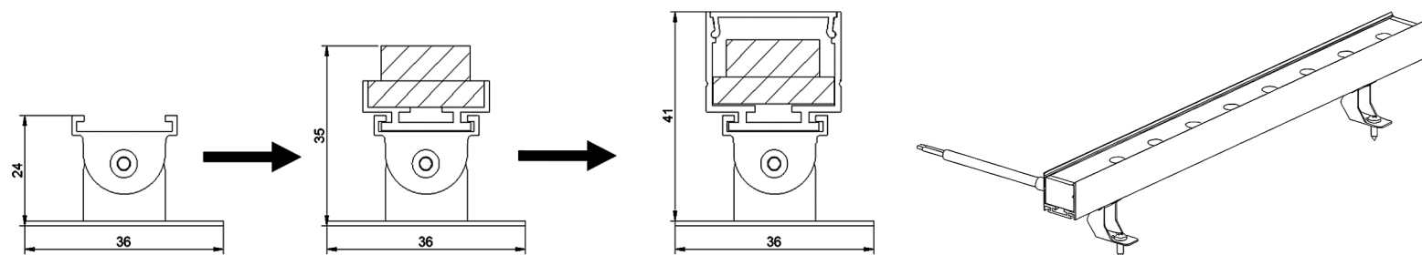
Rotatable bracket : 7022205-04
