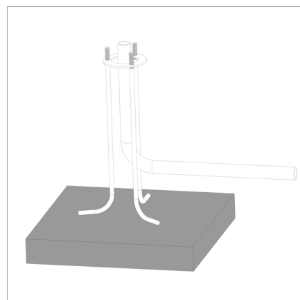
3. Install the conduit tube
